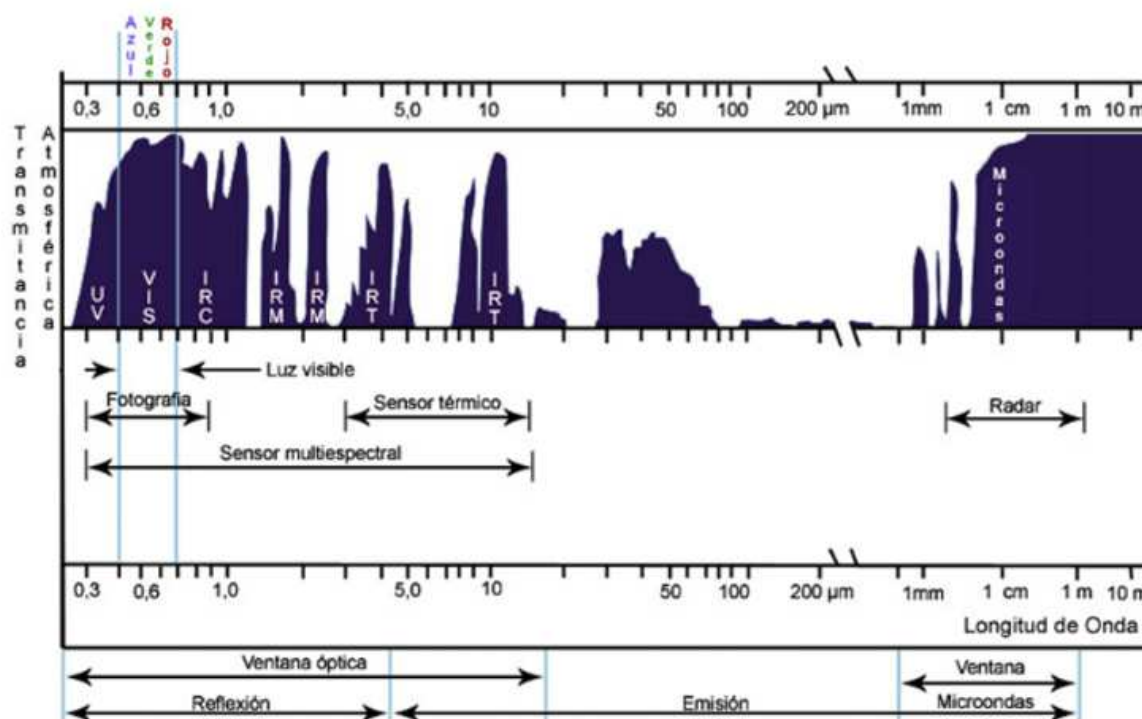
Fig. 3.- Espectro de radiación electromagnética
