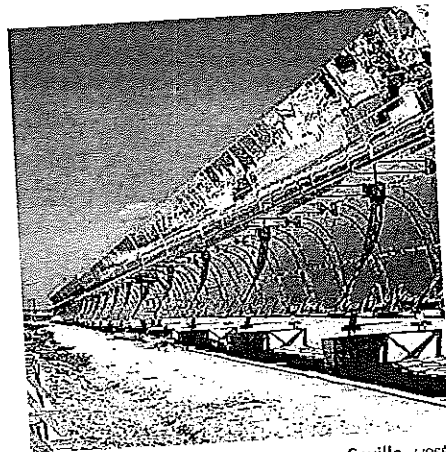
La Plataforma Solúcar de Abengoa en Sevilla. / JOSÉ ÁNGEL GARCÍA
