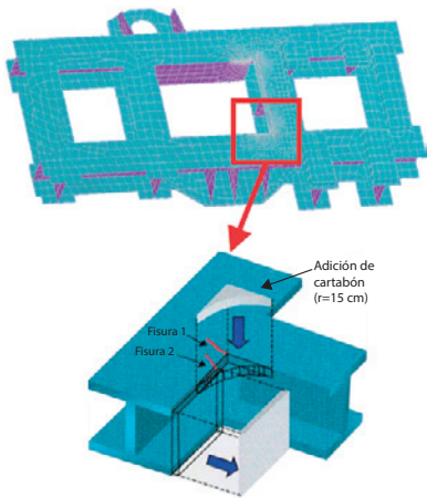
a) Modelo de elementos finitos de chasis de aerogenerador y propuesta de modificación
