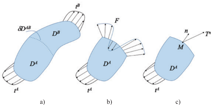
Figura 7. Hipótesis fundamental de la mecánica de los medios continuos sobre un ejemplo bidimensional
