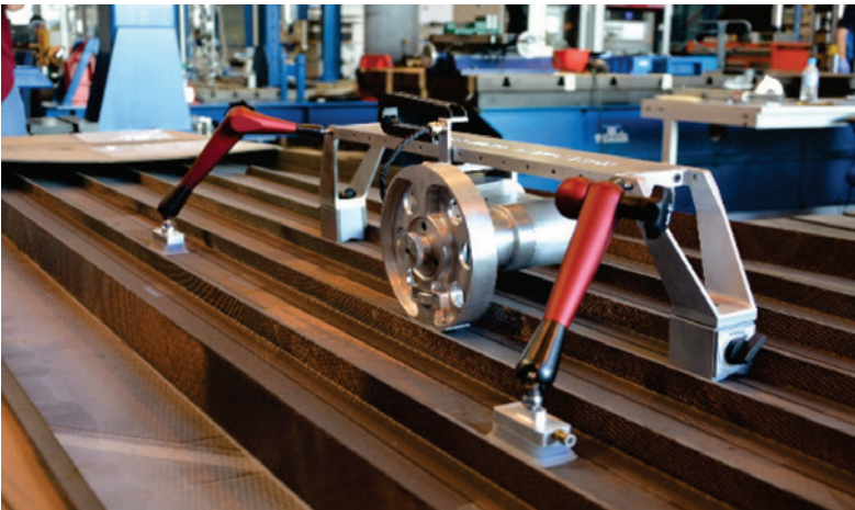
Figura 35. Dispositivos para la medida in situ de propiedades de un componente aeronáutico tras su fabricación
