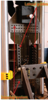
e) Ensayo y modelo de elementos finitos de un componente con «run-out»
