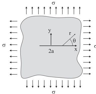
Figura 24. Grieta en medio infinito bajo cargas de tracción
