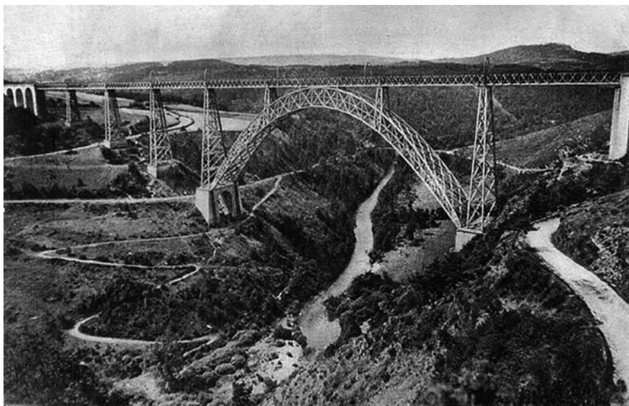
Figura 13. Viaducto de Garabit (1879-1885)
