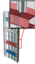
f) Ensayo y modelo de elementos finitos de un panel curvo a compresión
