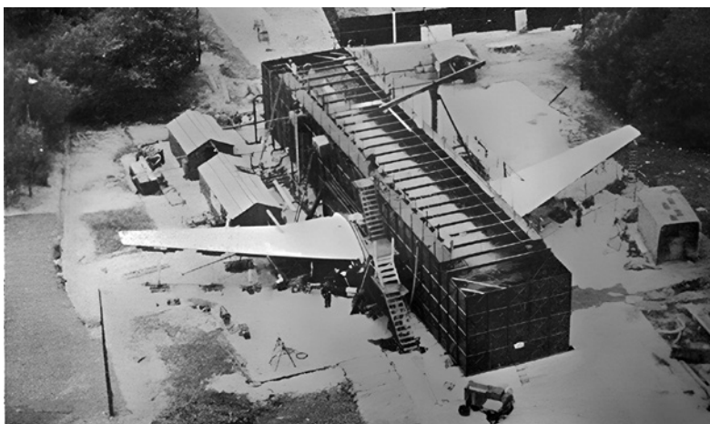
Figura 22. Ensayo a fatiga de un avión Comet en Farnborough
