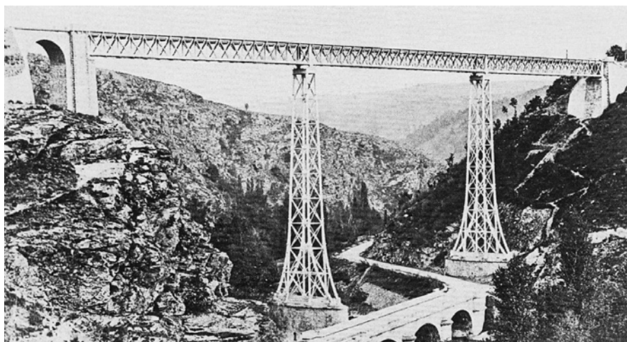
Figura 11. Viaducto de la Sioule (1869)
