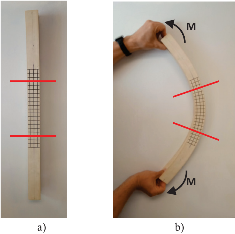
Figura 6. Ilustración de la hipótesis de Navier de secciones planas en un caso de flexión pura sobre una barra en forma de doble T: a) configuración indeformada, b) configuración deformada
