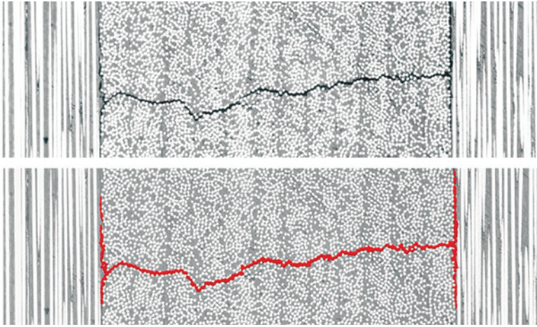
Figura 34. Grieta transversal en la lámina de 90 grados más daño entre láminas referenciable como grieta de delaminación para un laminado [0_{12}, 90_{12}, 0_{12}] (imagen obtenida en el laboratorio del GERM)
