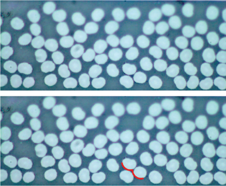
Figura 33. Despegues aislados en la lámina de 90 grados en un laminado cross-ply [0_{12}, 90, 0_{12}] (imagen obtenida en el laboratorio del GERM)
