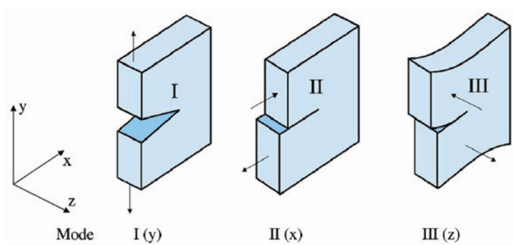
Figura 26. Modos de trabajo y propagación de una grieta
