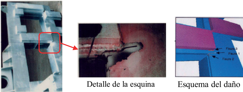
Figura 25. Daño en chasis de aerogenerador, estudiado y resuelto en el GERM
