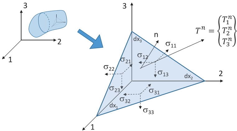
Figura 8. Equilibrio de un tetraedro infinitesimal (París[4])
